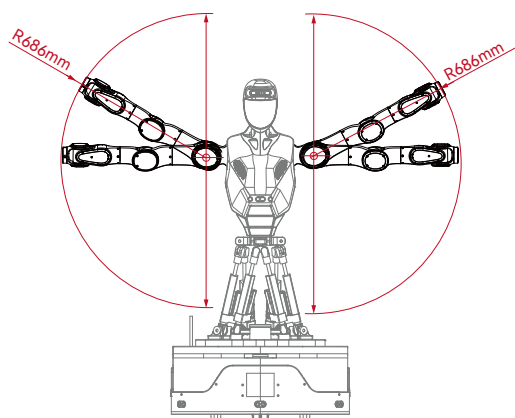
臂展尺寸
